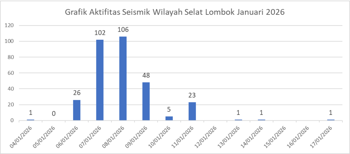
Gambar 4. Grafik Aktivitas Gempabumi Swarm Wilayah Selat Lombok Bulan Januari 2026
