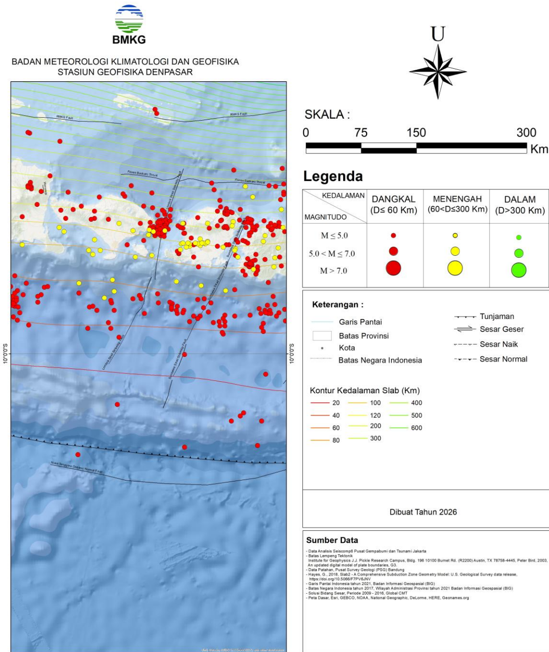
Gambar 3. Peta seismisitas Bali dan sekitarnya periode Januari 2026
